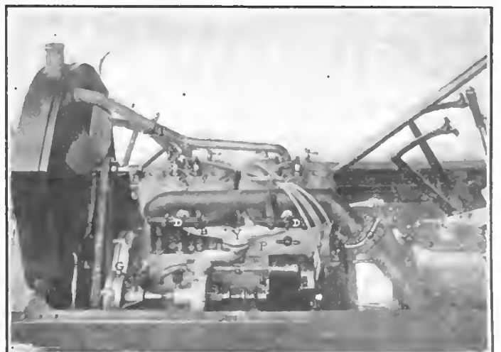
Fig. 3—The compact valve side of the G. J. G. motor
